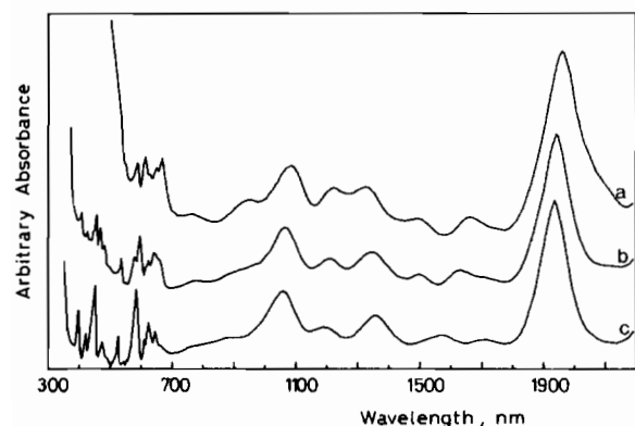
Fig. 2. Solid reflectance spectra of a, UI_4(\text{tbso})_2 ; b, U\text{Br}_4(\text{tbso})_2 ; c, U\text{Cl}_4(\text{tbso})_2 .
